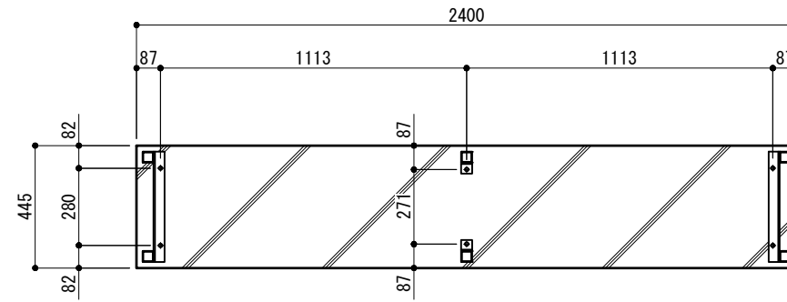
基礎伏図 S = 1 : 25
