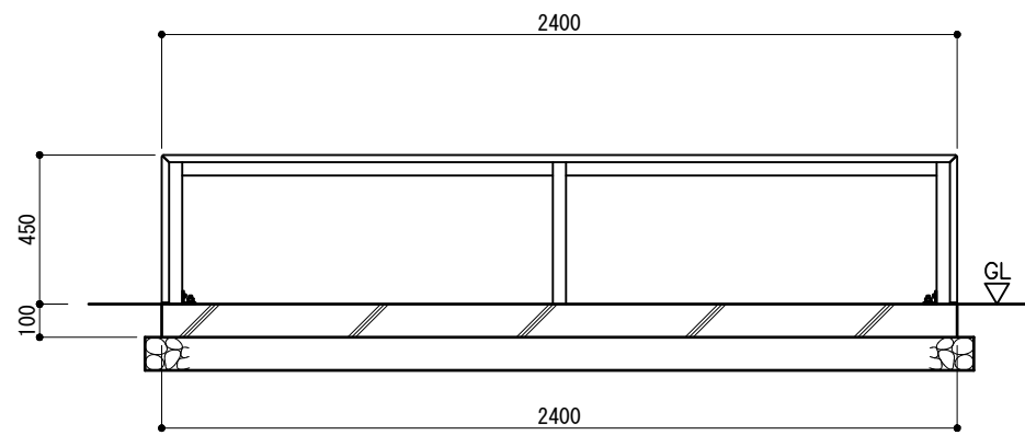
立面図 S = 1 : 25
